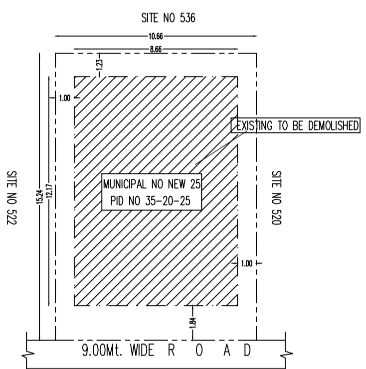
SITE PLAN (1:200)
